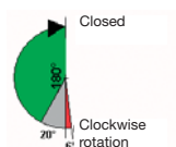
180° Actuator
